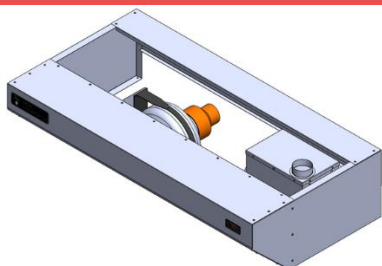
CAMPANA DE CONDENSACION -SISTEMA SIN SALIDA DE HUMO
